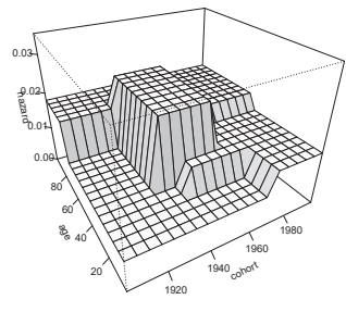
(d) Piecewise constant true hazard – perspective
