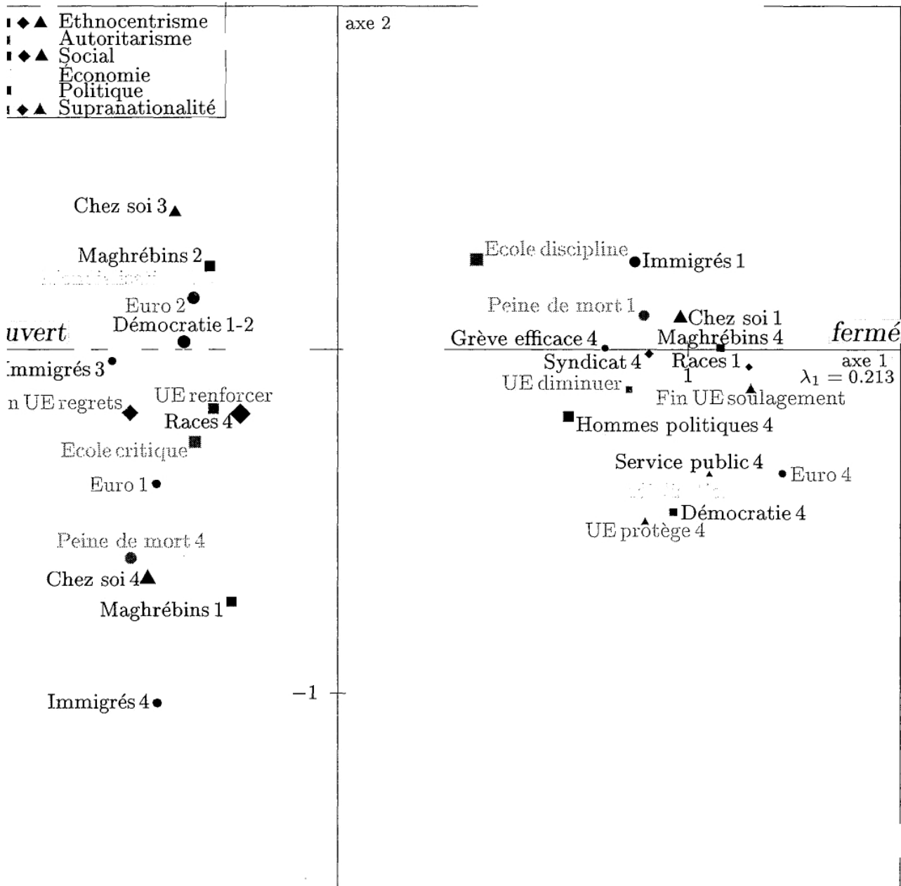
Graphique 1. Nuage des modalités dans le plan 1-2 : interprétation de l'axe 1
