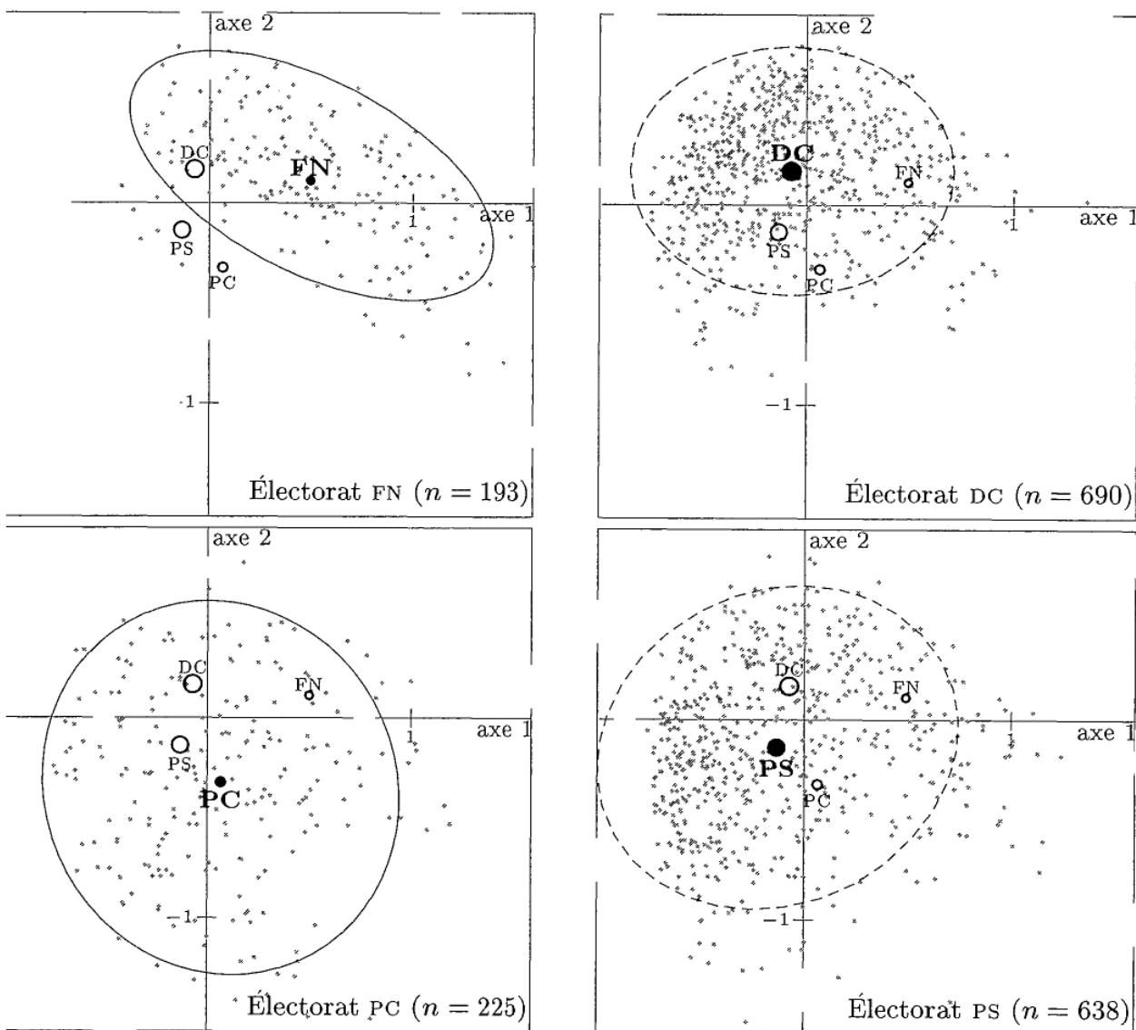
Plan 1-2 : ellipses de concentration avec leurs centres (cercles pleins) et les points moyens des autres électorats (cercles vides).
