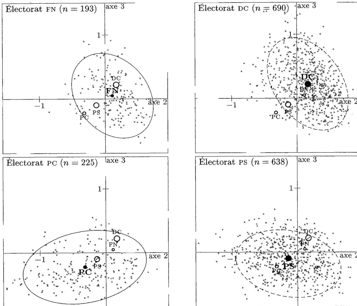
Plan 2-3 : ellipses de concentration avec leurs centres (cercles pleins) et les points moyens des autres électorats (cercles vides).
