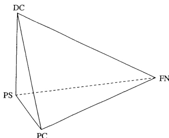
Graphique 6. Les 4 points moyens dans l'espace à 3 dimensions
