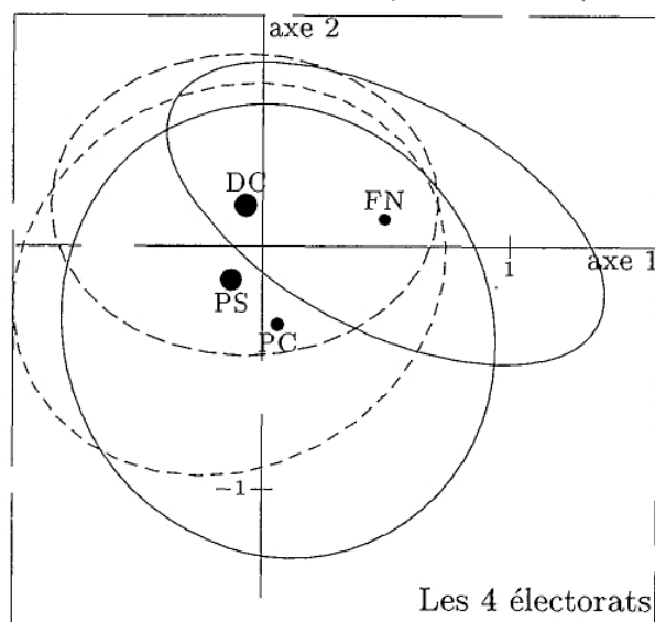
Ellipses de concentration des 4 électorats avec leurs centres.
