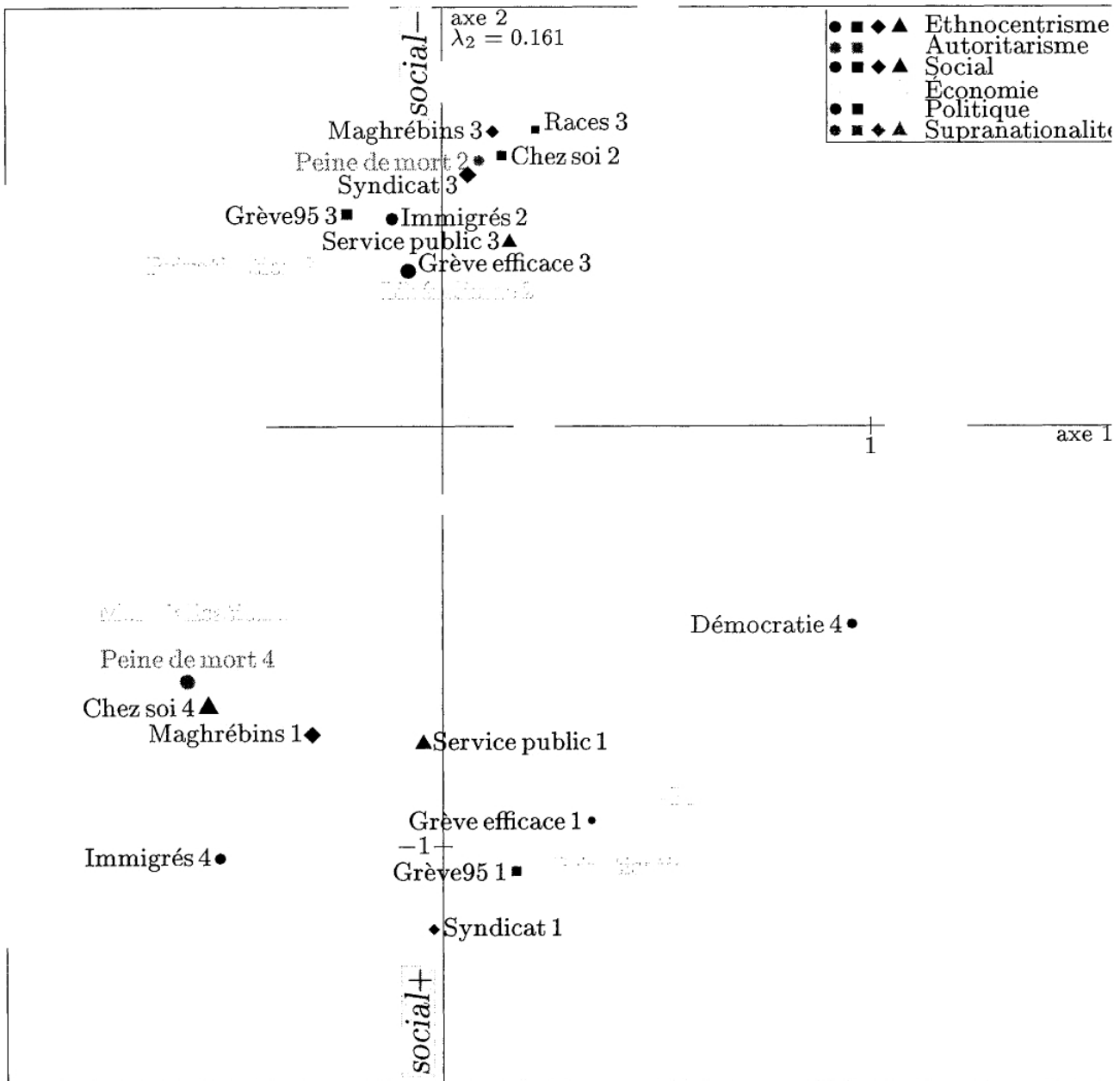
Graphique 2. Nuage des modalités dans le plan 1-2 : interprétation de l'axe 2
