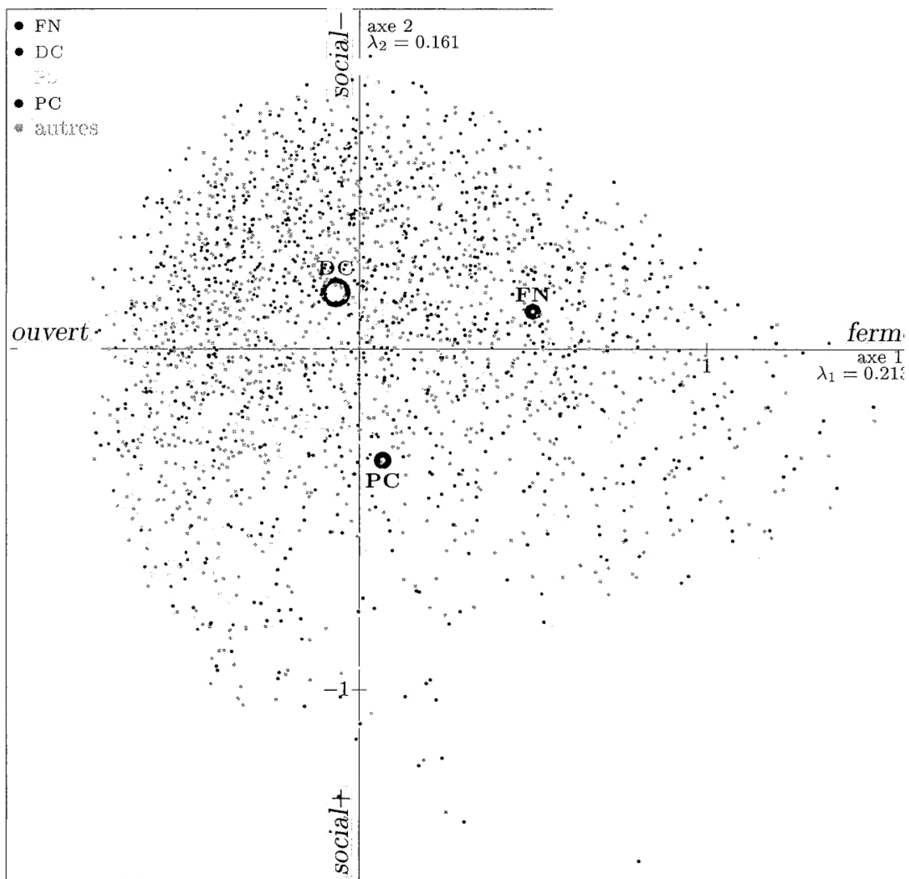
Graphique 4. Plan 1-2 Nuage des 2 980 individus marqués selon leurs votes et les 4 points moyens des électorats FN, DC, PS, PC
