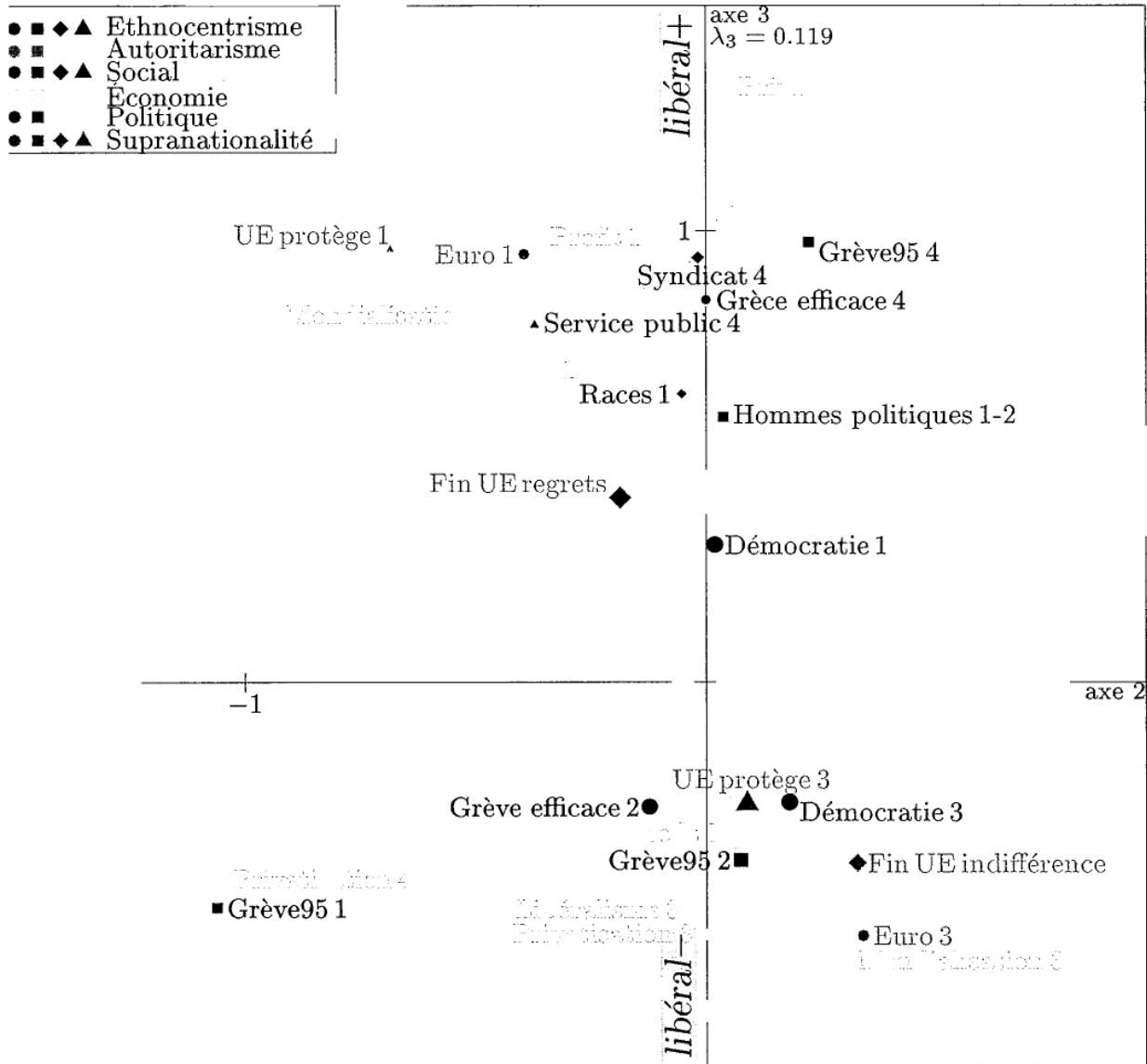
Graphique 3. Nuage des modalités dans le plan 2-3 : interprétation de l'axe 3
