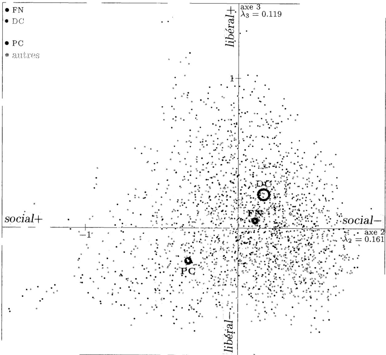
Figure 5. Plan 2-3 — Nuage des 2 980 individus marqués selon leurs votes et les 4 points moyens des électorats FN, DC, PS, PC
