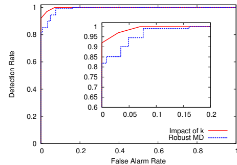
Fig. 17: ROC
