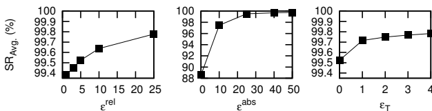
(d) Average suppression ratio for the combinations above.
