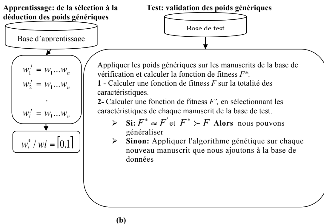
Figure 4.6. (a) Caractérisation et sélection de caractéristiques par algorithme génétique combiné à la coloration de graphes, (b) déduction des poids et test de validité du système
