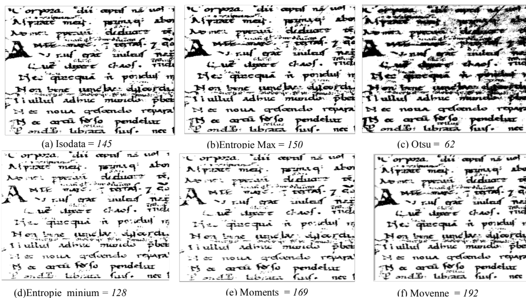
Figure 3.2. Résultats de binarisation avec un seuil global de binarisation: (a) Isodata (Velasco, [1980]), (b) Entropie Max (Cheng et al. [1998]), (c) Otsu (Otsu, [1979]), (d) Entropie minimum (Li et Lee, [1993]), (e) Moments (Tsai, [1985]), (f) Moyenne (Glasbey, [1993])
