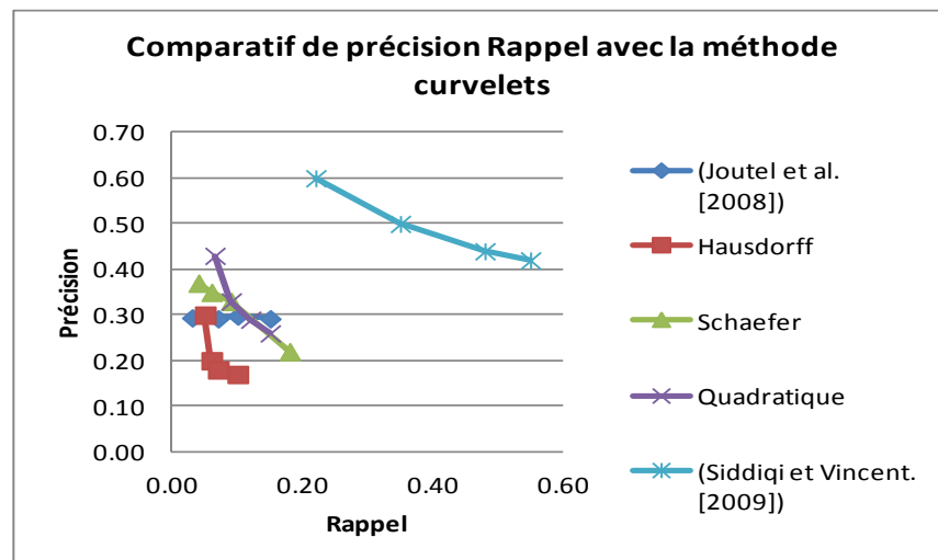
Figure 5.4. Courbes de précision-rappel, base IRHT
